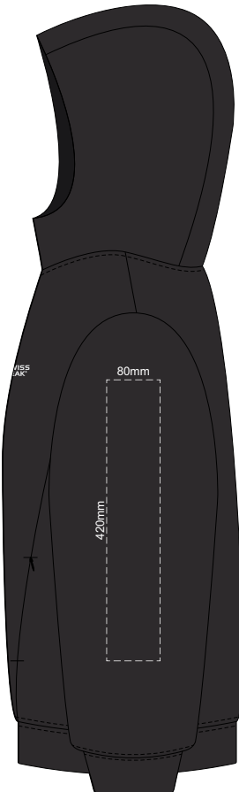
3XL LEFT SLEEVE
